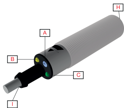
Fig. 1 CA18 Cable
